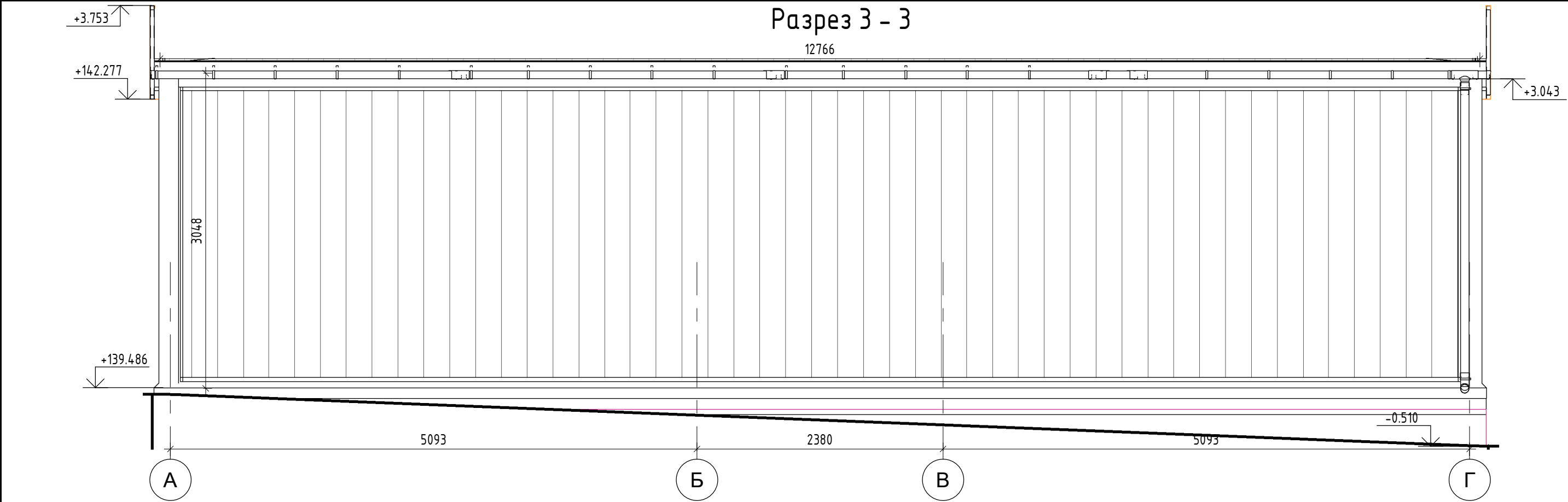
Разрез по задней части
