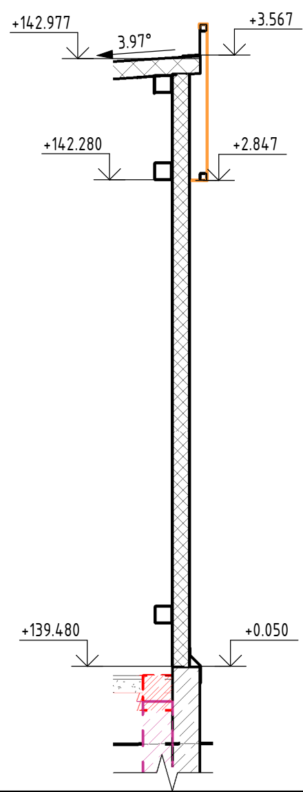
Разрез по фасадной части
