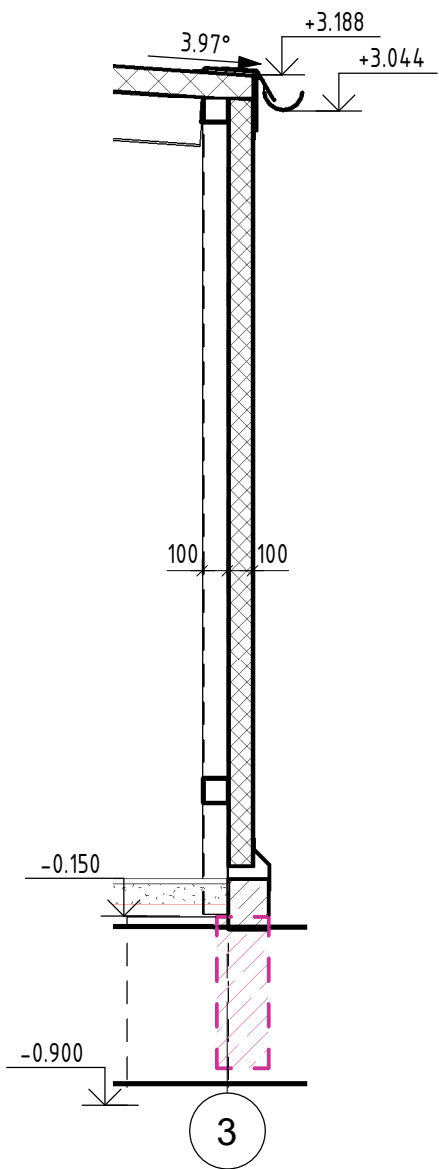
Разрез по задней части
